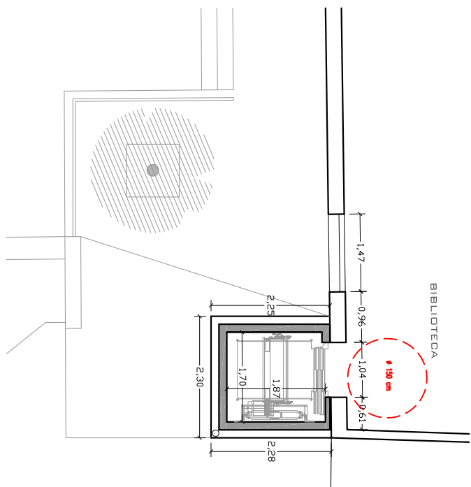
PLANTA SEGONA PROPOSTA - E 1:100
